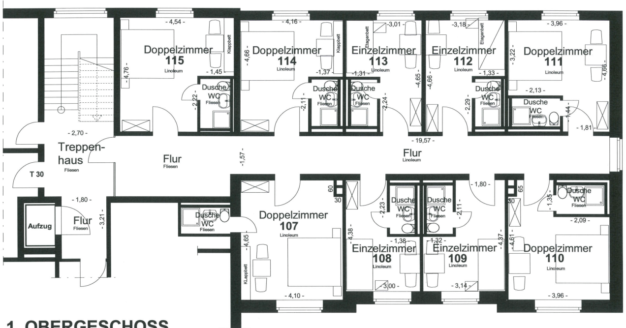
1. OBERGESCHOSS
