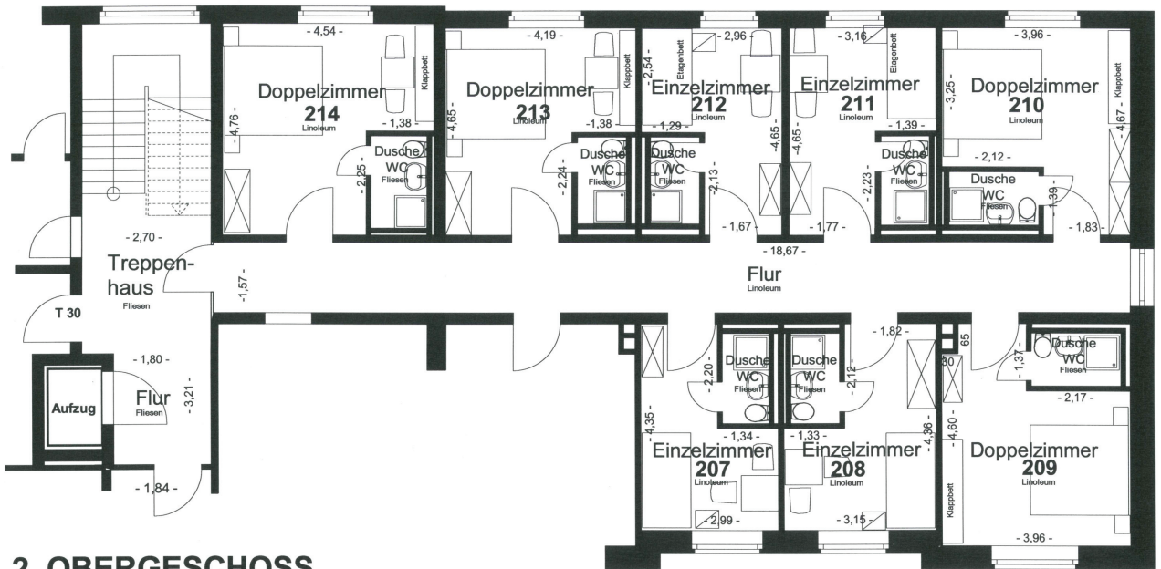
2. OBERGESCHOSS
