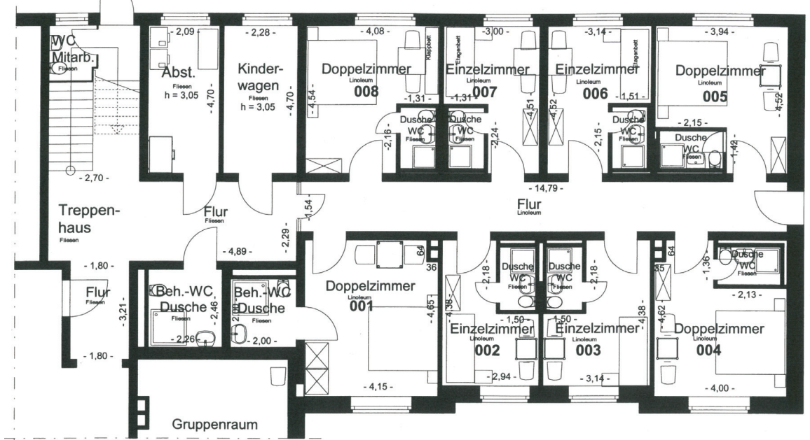
ERDGESCHOSS
